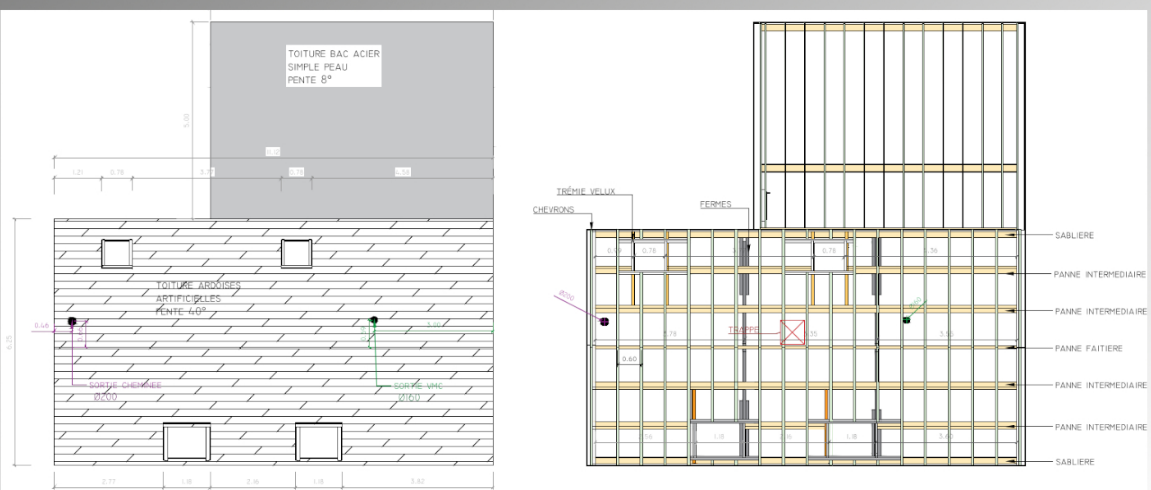
Plans de toiture
