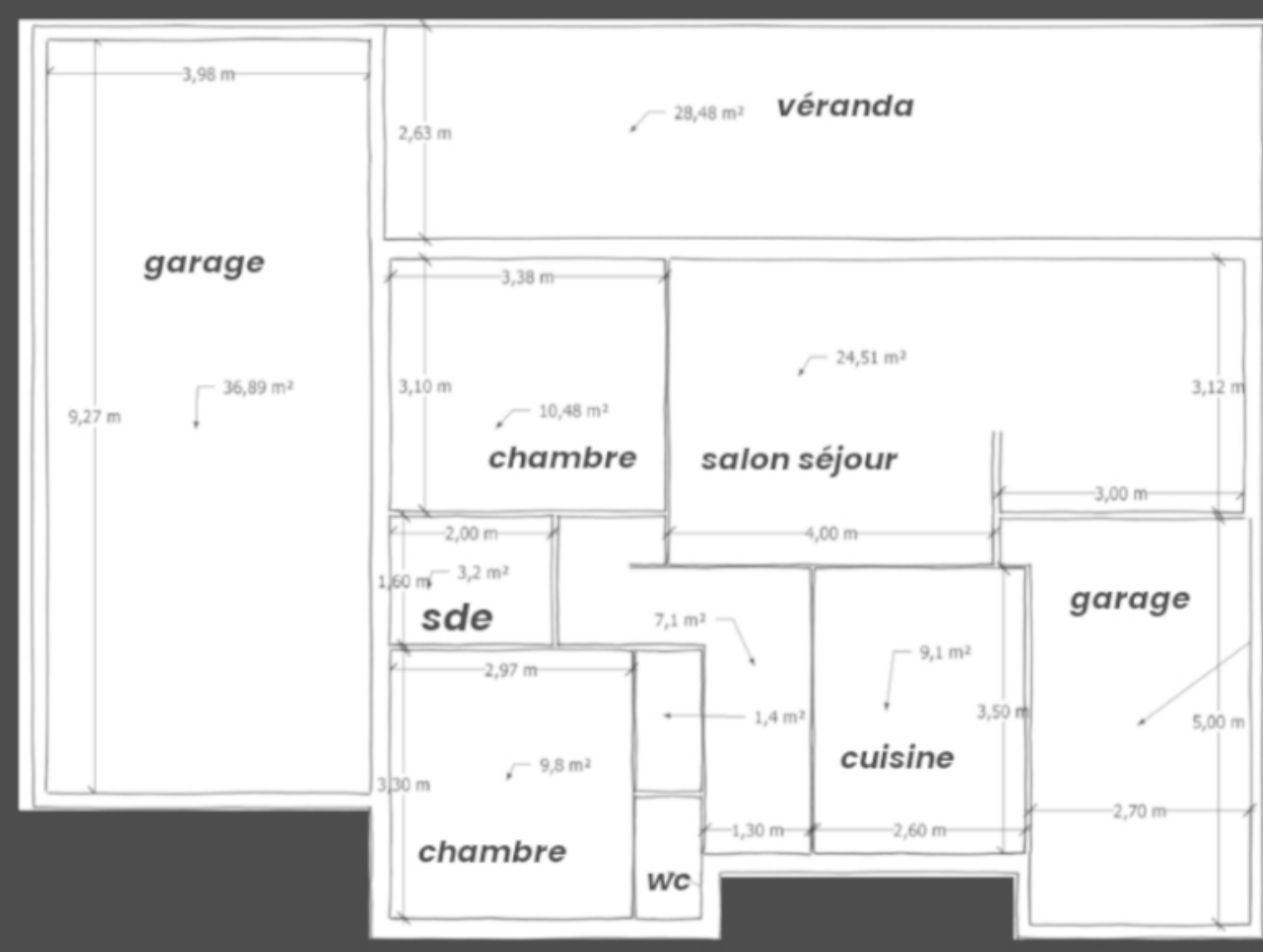
Plan état existant
