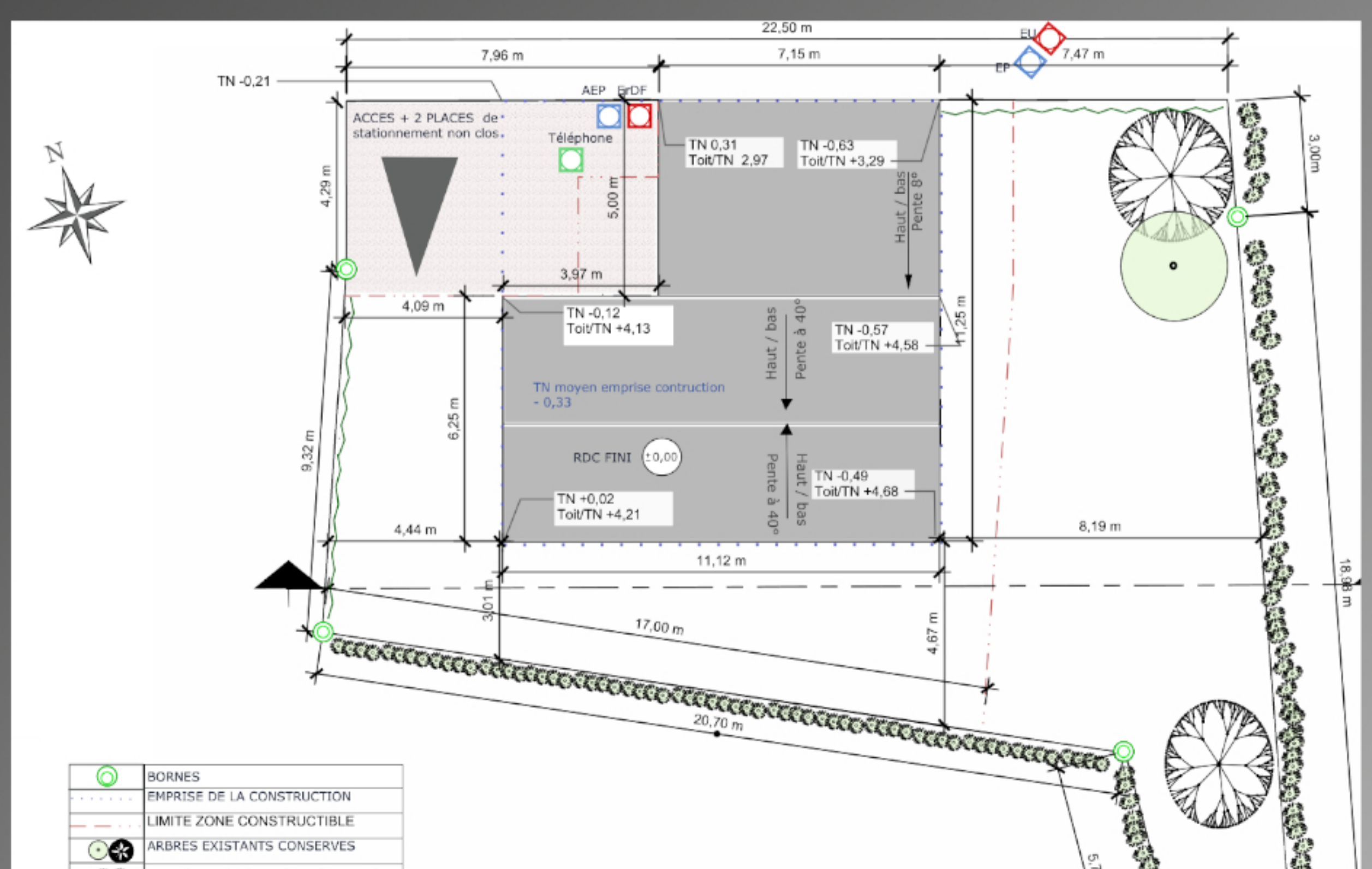
Plans de masse
